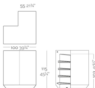
VELA Barra Esquina VELA Corner Bar
